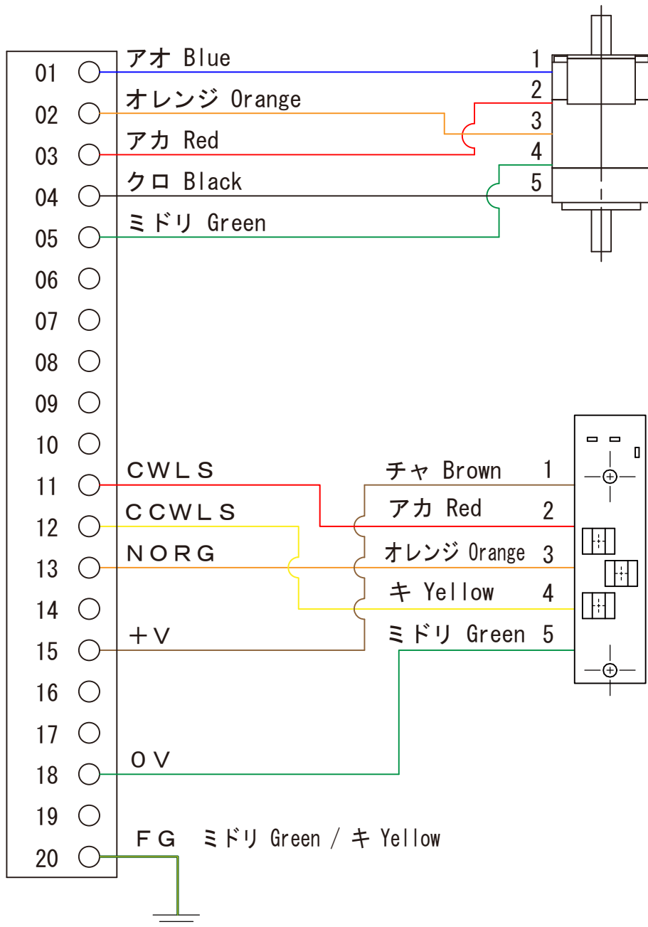
フォトセンサ基板 Photosensor Circuit Board F-116
